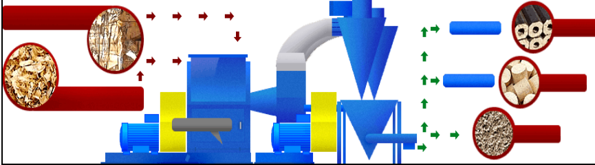
Фиг. 1. Принципна схема на инсталация за производство на брикети или пелети
